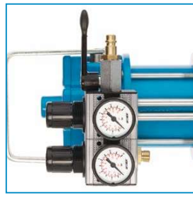
Doppeldruckluftregler für Spritzdruck und Zerstäuberluft (Air Combi)
